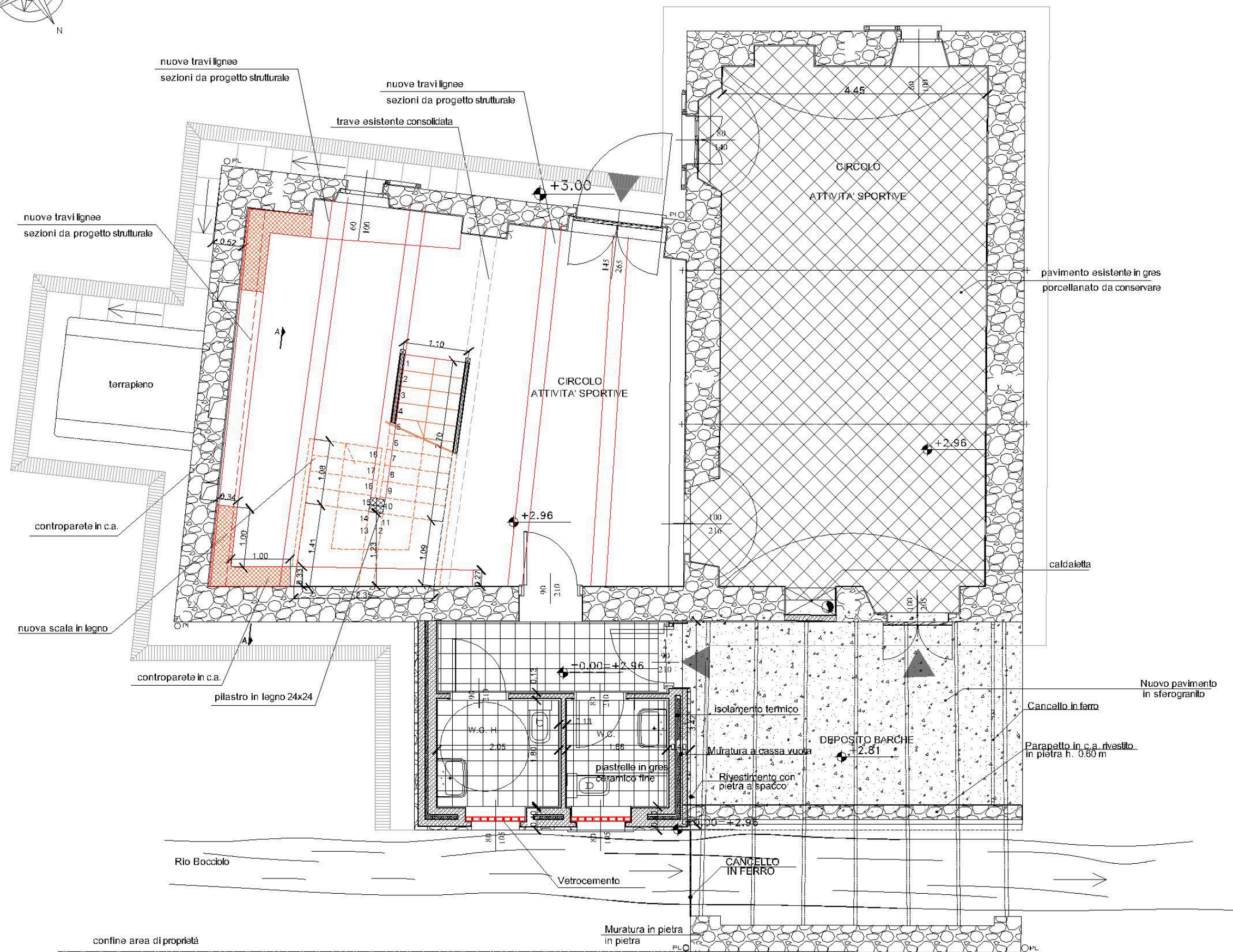
Pianta piano terra - controparete in c.a. - travi lignee solaio - dettaglio scala in legno Scala 1:50
